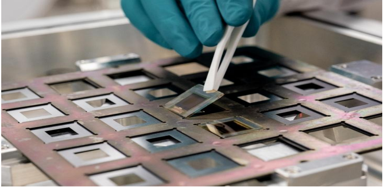
चित्र 7: प्रयोगशाला में निर्मित पेरोव्स्काइट सौर कोशिका की सूक्ष्म संरचना। पेरोव्स्काइट कोशिकाओं में ABX_3 क्रिस्टल संरचना (जहाँ A = CH_3NH_3^+/Cs^+ , B = Pb^{2+}/Sn^{2+} , X = I^-/Br^-/Cl^- ) का उपयोग प्रकाश अवशोषक परत के रूप में किया जाता है। इनका बैंड गैप (1.2-2.3 eV) समायोज्य होता है [9]
