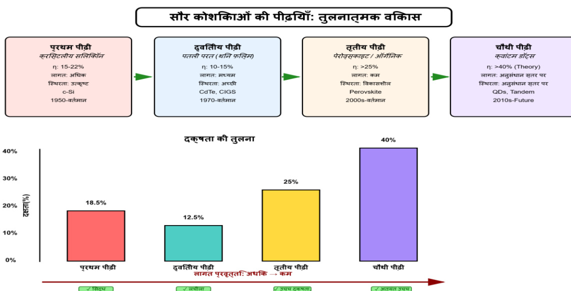
चित्र 6: सौर कोशिकाओं की चार पीढ़ियों का तुलनात्मक विश्लेषण: प्रथम पीढ़ी (c-Si, 15-22%) से चौथी पीढ़ी (क्वांटम डॉट/टैंडम, सैद्धान्तिक >40%) तक का विकास क्रम [4]
