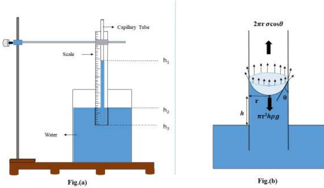
चित्र 2 (a) केशिका क्रिया (capillary action) का चित्रण, (b) बल संतुलन से केशिका में द्रव का ऊपर चढ़ना (capillary rise)
