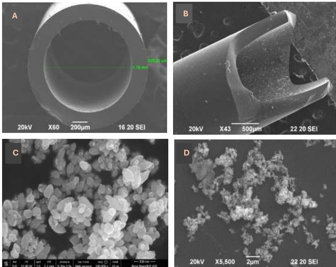
चित्र 8: FESEM विश्लेषण (A) 200 \mu m पर (B) 500 \mu m पर (C) 500nm पर (D) 2 \mu m पर (यह चित्र संदर्भ 51 के डाटा को उपयोग कर दुबारा से बनाया गया है)
