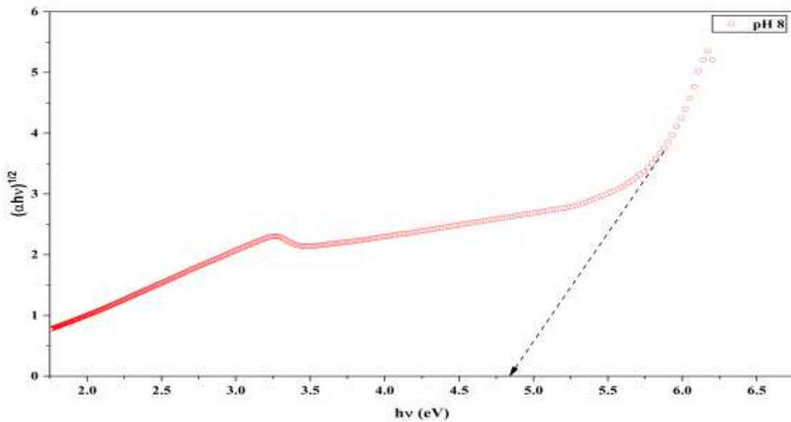
चित्र 6: इनडायरेक्ट ट्रांज़िशन के लिए ZnO नैनोपार्टिकल्स का टॉस प्लॉट (Tauc plot) (यह चित्र संदर्भ 51 के डाटा को उपयोग कर दुबारा से बनाया गया है)
