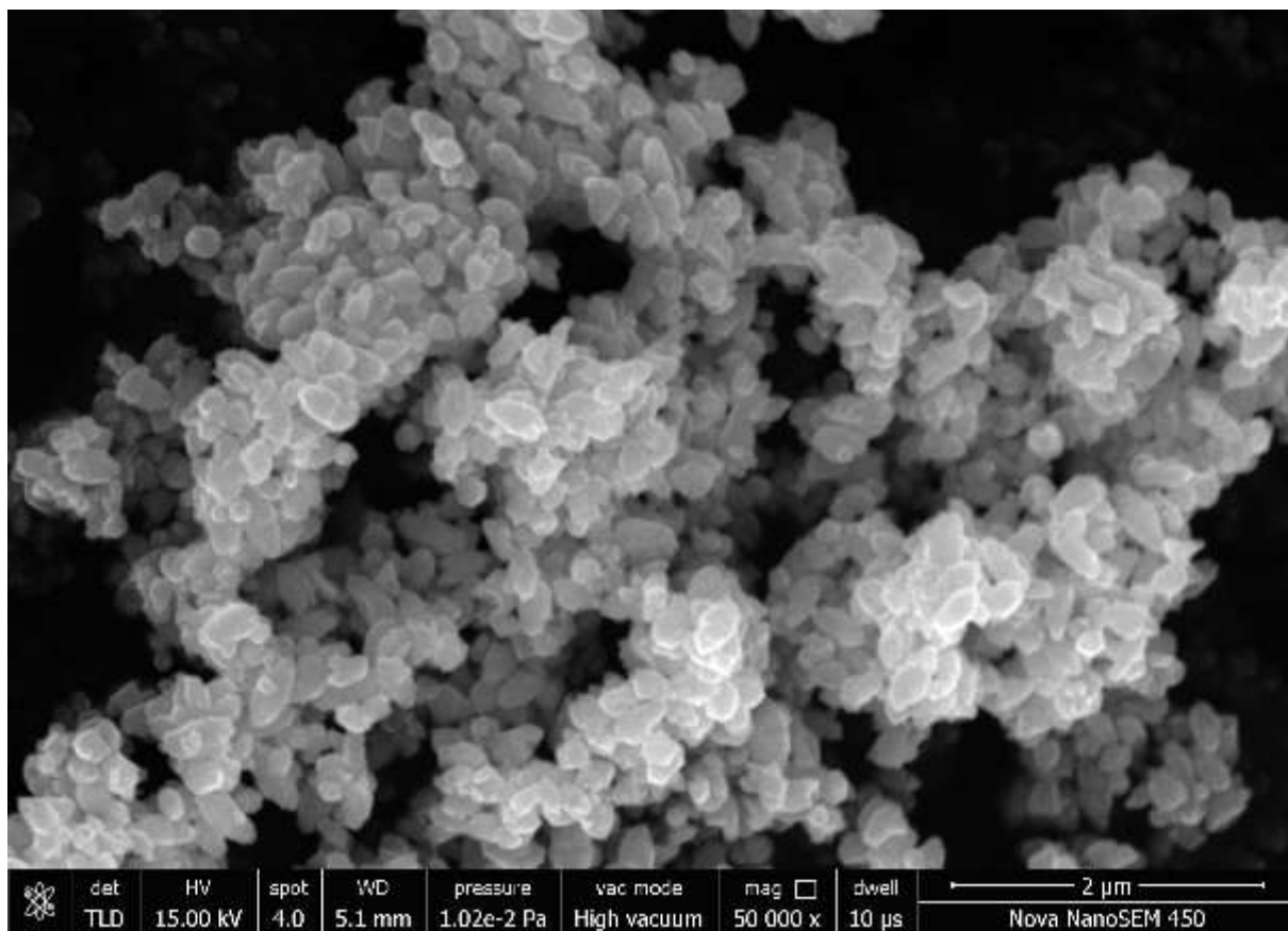
चित्र 13: यह चित्र जिंक ऑक्साइड (ZnO) नैनोकण का SEM (स्कैनिंग इलेक्ट्रॉन माइक्रोस्कोपी) इमेज दर्शाता है।
