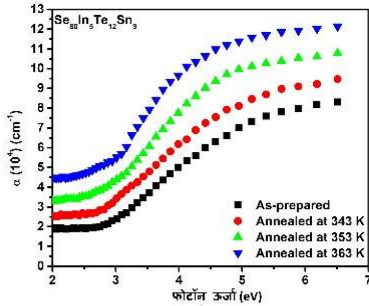
चित्र 4: \text{Se}_{80}\text{In}_5\text{Te}_{12}\text{Sn}_9 नैनो चैल्कोजेनाइड की प्रारंभिक और एनीलड पतली फिल्मों के आपतित फोटॉन ऊर्जा ( h\nu ) के साथ अवशोषण गुणांक ( \alpha ) में परिवर्तन का ग्राफ।
