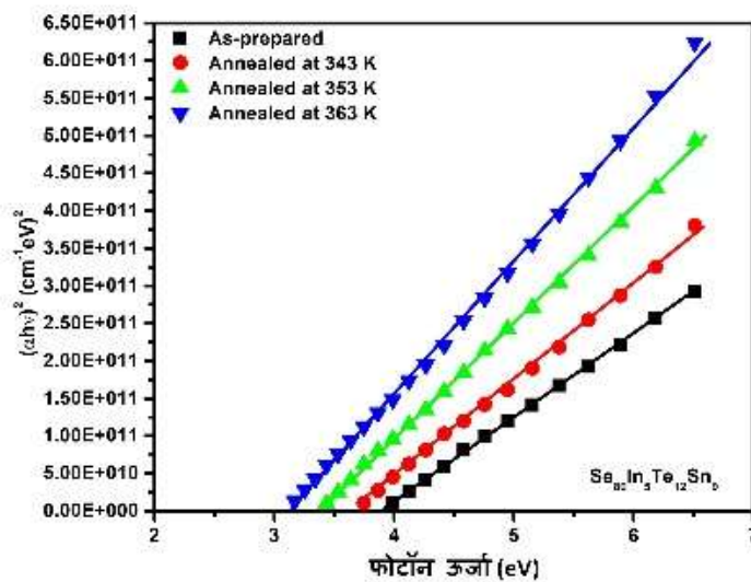
चित्र 5: \text{Se}_{80}\text{In}_5\text{Te}_{12}\text{Sn}_9 नैनो चैल्कोजेनाइड की प्रारंभिक और एनीलड पतली फिल्मों के लिए ऊर्जा ( h\nu ) के साथ (\alpha h\nu)^2 का ग्राफ।
