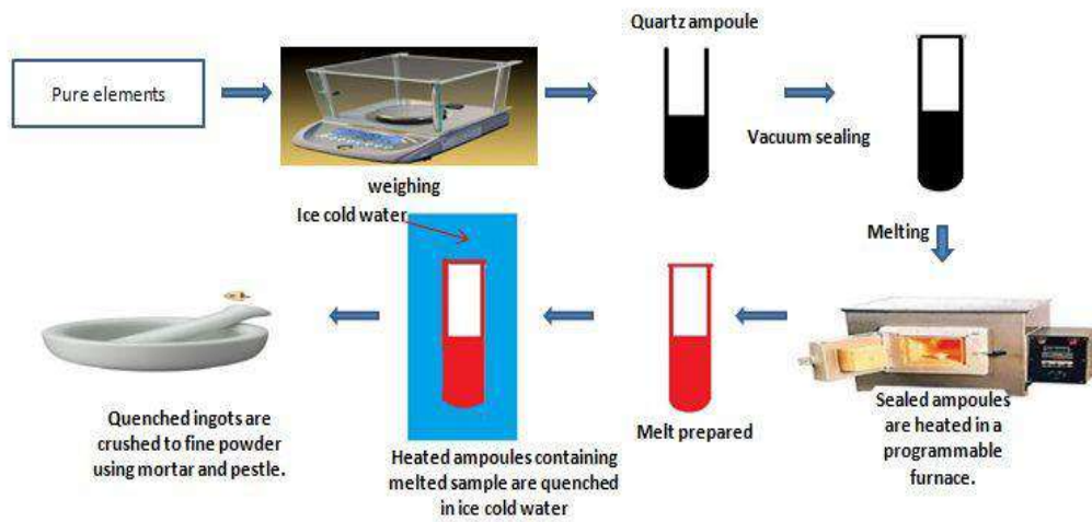
चित्र 1: बल्क चैल्कोजेनाइड ग्लास के संश्लेषण हेतु मेल्ट क्वेंचिंग तकनीक का योजनाबद्ध आरेख (यह चित्र सन्दर्भ संख्या [1] से लिया गया है)
