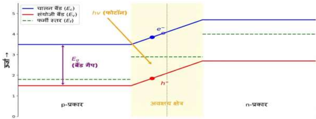
चित्र 2: पी-एन संधि का ऊर्जा बैंड आरेख: चालन बैंड ( E_c , नीला), संयोजकता बैंड ( E_v , लाल), फर्मी स्तर ( E_f , हरा), बैंड गैप ( E_g ), अवक्षय क्षेत्र (पीला छायांकित), तथा फोटॉन ( h\nu ) अवशोषण से इलेक्ट्रॉन-होल युग्म उत्पादन की प्रक्रिया दर्शायी गई है। (स्व-रचित आरेख)
