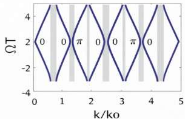
चित्र 2- फोटोनिक टाइम क्रिस्टल में फ्रीक्वेंसी बैंड संरचना
